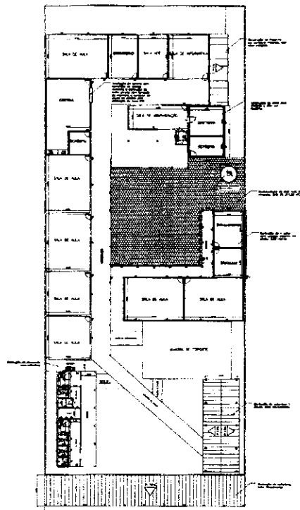
PLANTA BAIXA - AMPLIAÇÃO ESCOLA GERUSA LEITE
