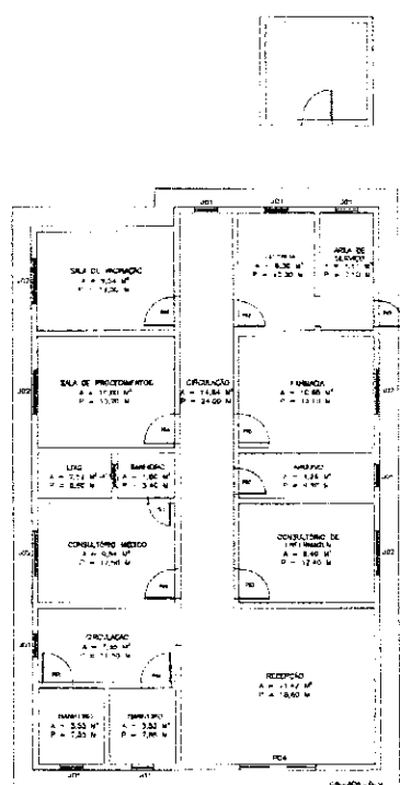
PLANTA BAIXA
