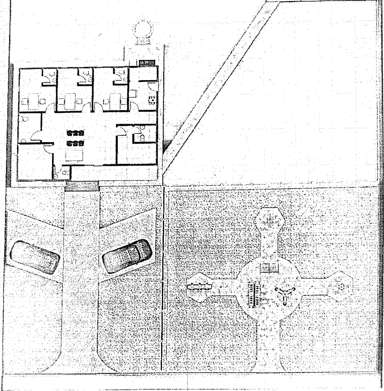
1 Planta Baixa Humanizada 1 : 200
