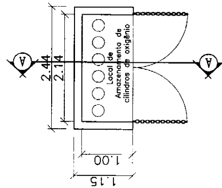
PLANTA BAIXA
