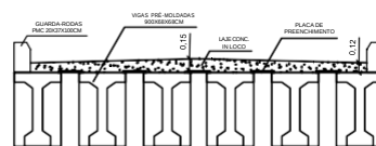
CORTE TRANSVERSAL - CC ESC.: 1/50
