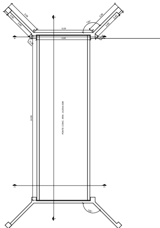
PLANTA BAIXA - PONTE 14,00x4,50M ESC.: 1/100
