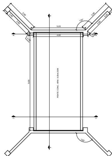
PLANTA BAIXA - PONTE 9,00x4,50M ESC.: 1/100
