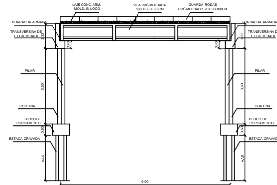
CORTE LONGITUDINAL - AA ESC.: 1/100
