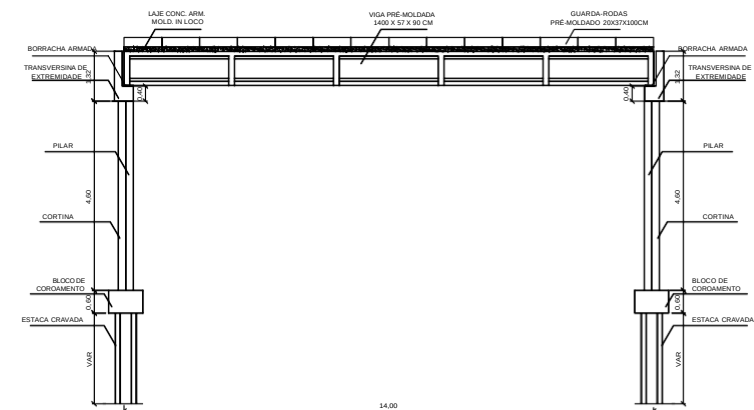
CORTE LONGITUDINAL - AA ESC.: 1/100
