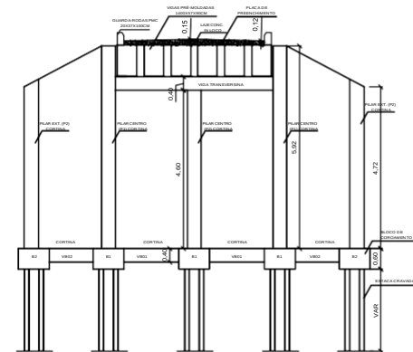
CORTE TRANSVERSAL - BB ESC.: 1/100
