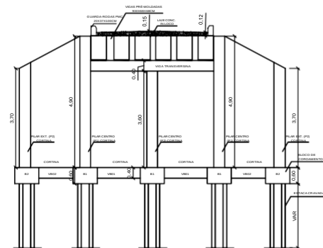
CORTE TRANSVERSAL - BB ESC.: 1/100
